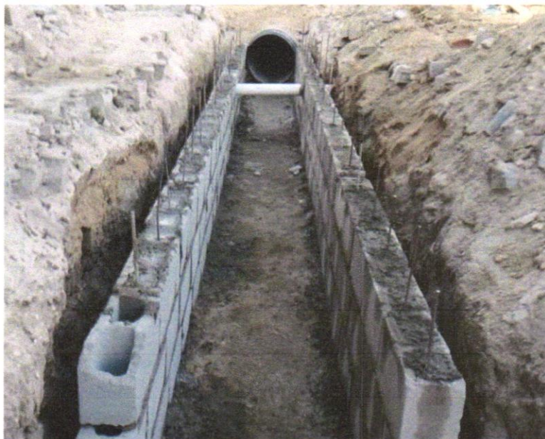
Foto 04 - ALVENARIA DE BLOCOS DE CONCRETO ESTRUTURAL 14X19X39 CM, (ESPESSURA 14 CM) FBK = 14,0 MPA, PARA PAREDES COM ÁREA LÍQUIDA MENOR QUE 6M 2 , SEM VÃOS, UTILIZANDO PALHETA. AF_12/2014
